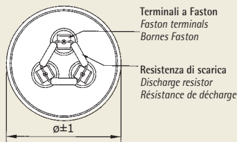
Tipologia terminali per Condensatori ø 60 mm Type of terminals for Capacitors ø 60 mm Type de bornes pour Condensateurs ø 60 mm
