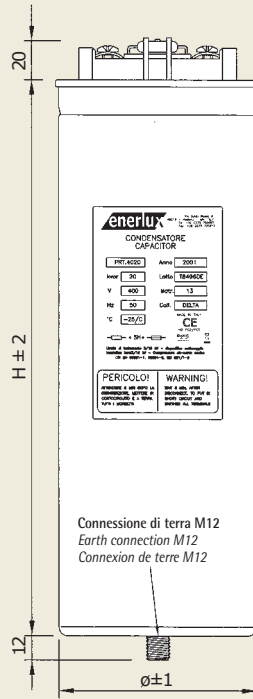
Tipologia terminali per Condensatori ø 75-85-100 mm Type of terminals for Capacitors ø 75-85-100 mm Type de bornes pour Condensateurs ø 75-85-100 mm
