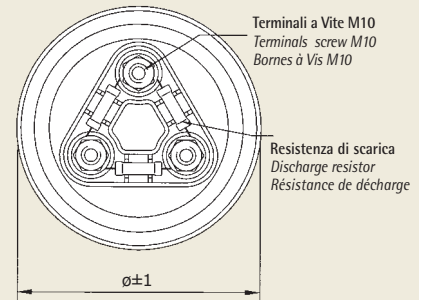
Tipologia terminali per Condensatori ø 120 mm Type of terminals for Capacitors ø 120 mm Type de bornes pour Condensateurs ø 120 mm
