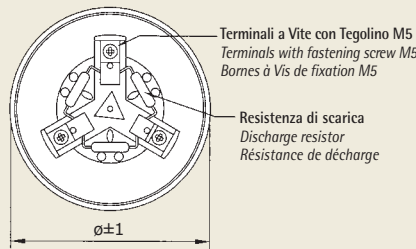
Tipologia terminali per Condensatori ø 75-85-100 mm Type of terminals for Capacitors ø 75-85-100 mm Type de bornes pour Condensateurs ø 75-85-100 mm
