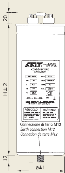
Tipologia terminali per Condensatori ø 60 mm Type of terminals for Capacitors ø 60 mm Type de bornes pour Condensateurs ø 60 mm
